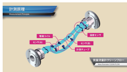
【計測原理】質量流量計クリーンフロー®
