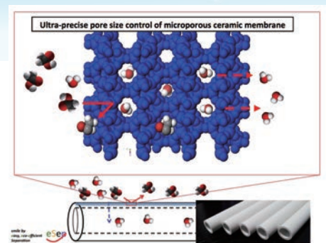
図1 ナノセラミック膜の分子分離の原理 細孔を超精密制御ができるため、分子の粒子径に合わせて分離が可能となる。
