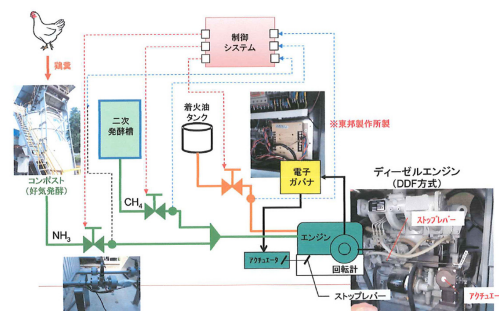
バイオガス発電システム 埼玉県セイメイファームでバイオガス発電実験プラントを実施中。
