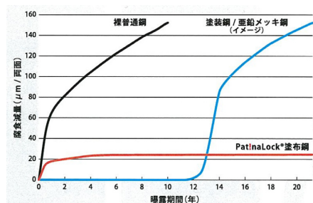
図2 裸普通鋼、塗装鋼/亜鉛メッキ鋼、Pat!naLock®塗布鋼の曝露期間と腐食の進行具合の関係
