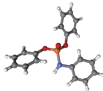
「ビゴールFV」シリーズに使用されているADPP(アニリノジフェニルホスフェート)
