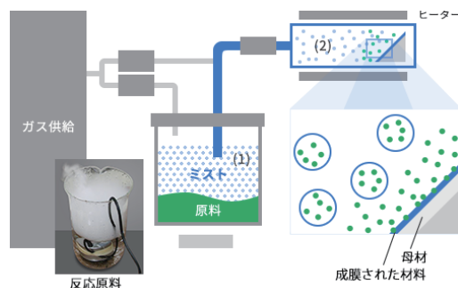
図2 ミストCVDの基本的な原理 液中の原料成分が、超音波でミスト状となり、ガス化したのち加熱した母材上で成膜・結晶化させるプロセス
