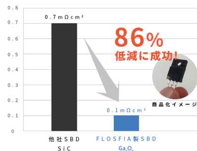
図1 試作したSBDの従来技術との比較 従来型と比べて約9割程度オン抵抗を低減
