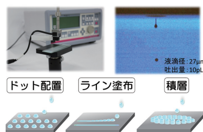
図3 吐出応用例
